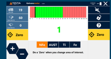
Galvanometer
